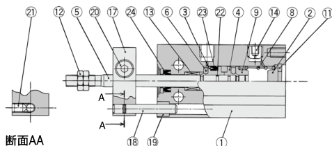
断面AA
