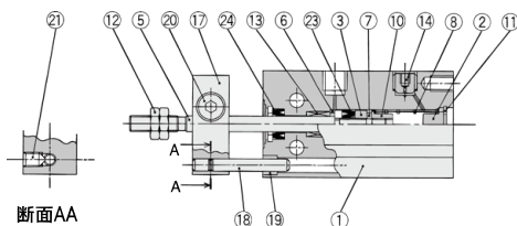
断面AA
