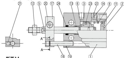
断面AA
