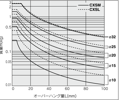
グラフ 11 V = 400mm/s超 ~10st
