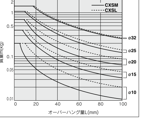
グラフ 12 V ~ 400mm/s ~30st
