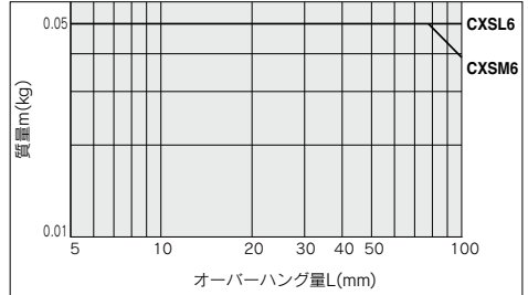
グラフ② V=300(mm/s)
