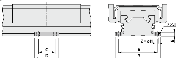
サイドサポートB MY-S□B
