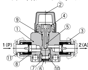
3ポート弁/VHK3Aシリーズ
