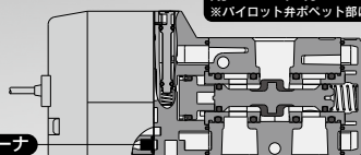
ストレーナ
