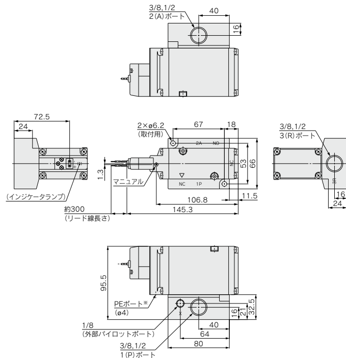
グロメツ(G) DC仕様ランプ・サージ電圧保護回路 なしの場合
