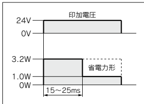
〈省電力形電力波形〉(定格電圧24VDC時)
