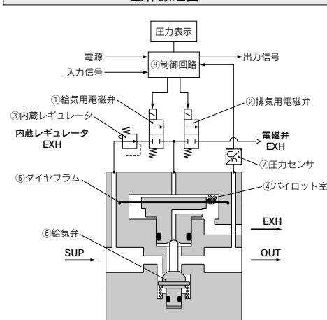
動作原理図
