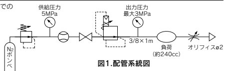
図1.配管系統図
