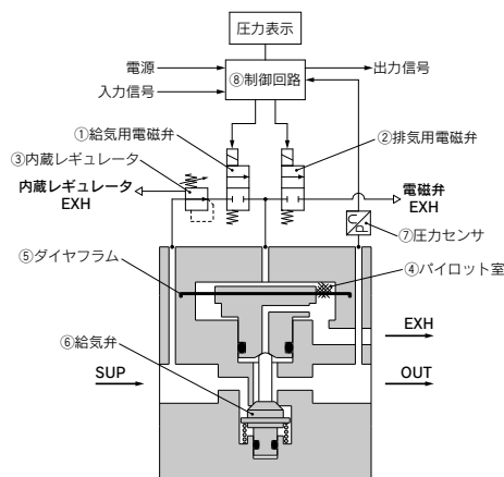
動作原理図
