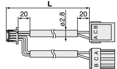
EX510-VW□Q
