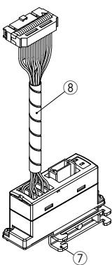
EX510-S□02C (Series SJ)
