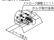
MY2H-A25L2-6N-XB20 (ショートスペーサのみ)
