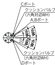
A-A' 矢視図
