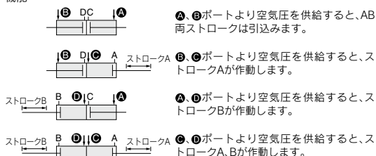
CJ2シリーズ
