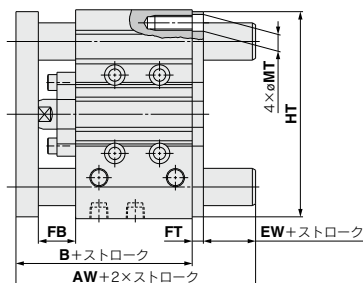
両側ルブリテナ付
