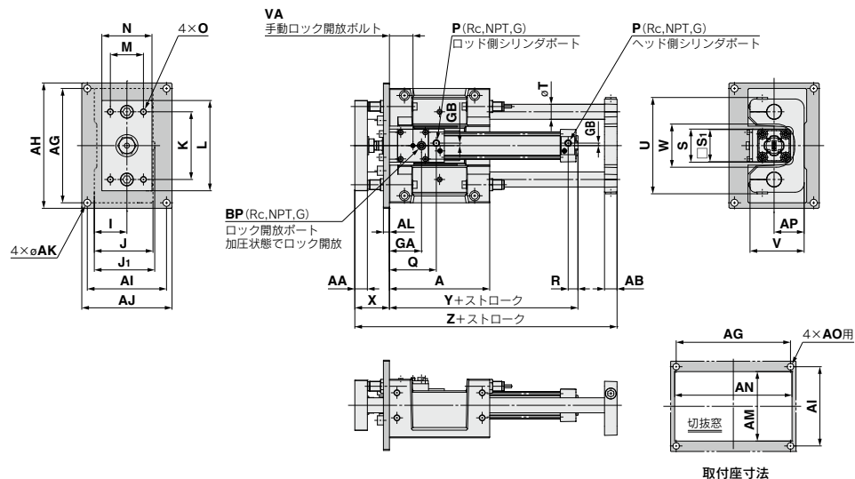
取付座寸法
