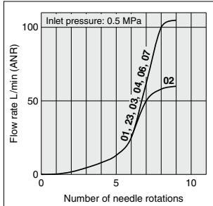
10-AS1□□1FSG□-M5, 10-AS1□11FSG□-M5
