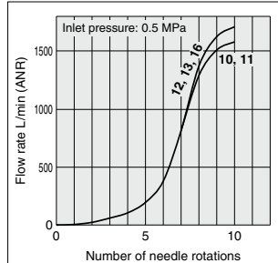
10-AS4□□1FSG□, 10-AS4□11FSG□
