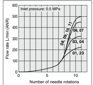
10-AS2□□1FSG□-02, 10-AS2□11FSG□-02
