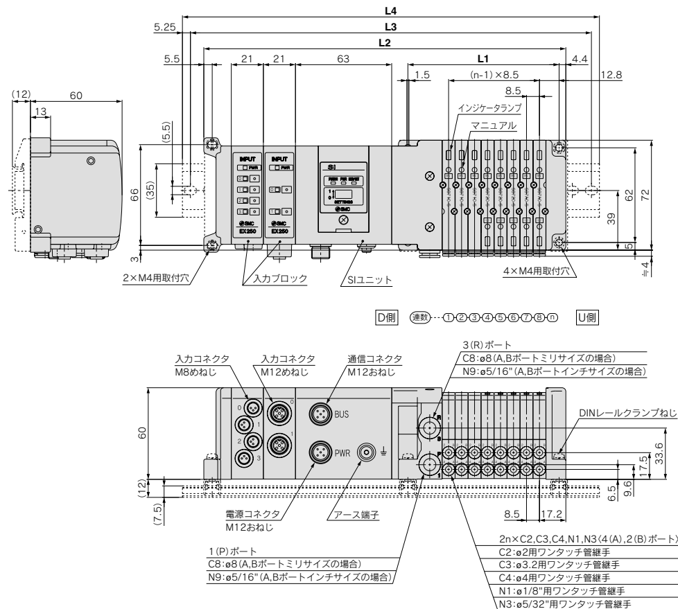
寸法表
