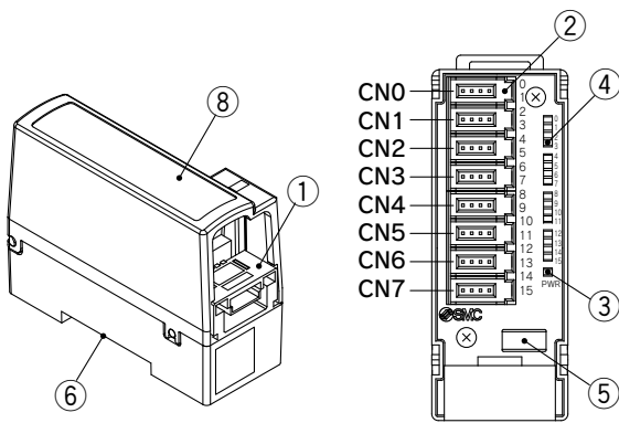
カバーを取外した状態
