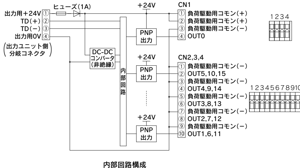
端子台コネクタ (CN1)
