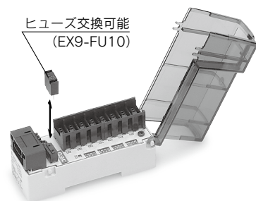
1コネクタ2入力タイプ
