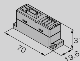
EX510シリーズ
