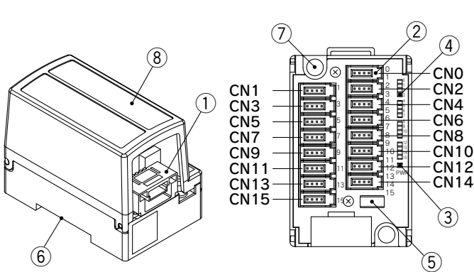
カバーを取外した状態
