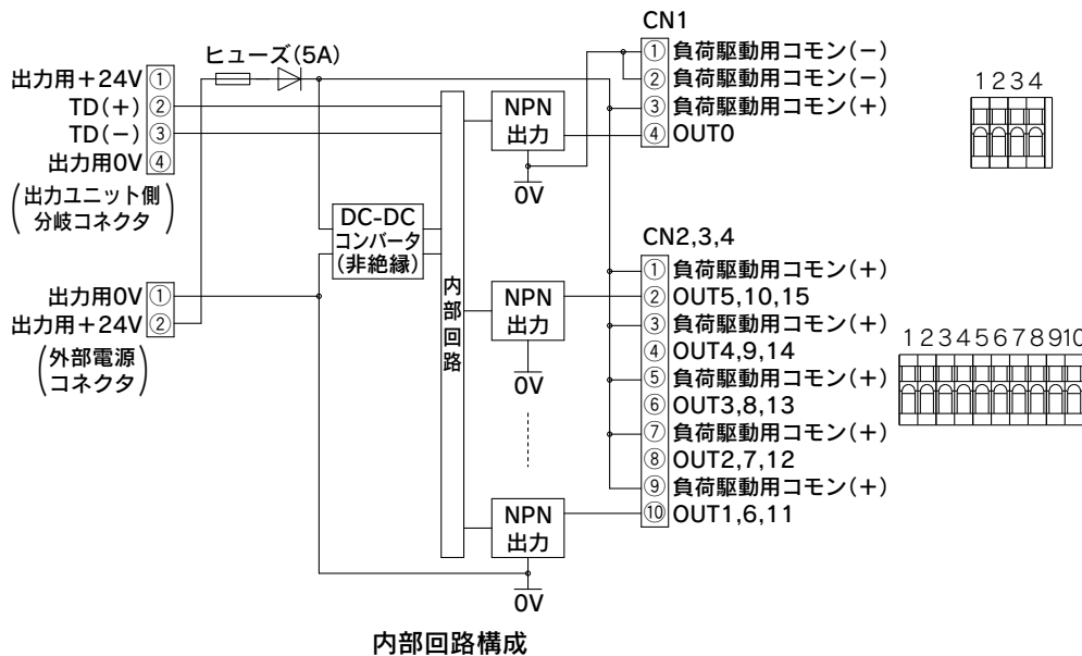
端子台コネクタ (CN1)
