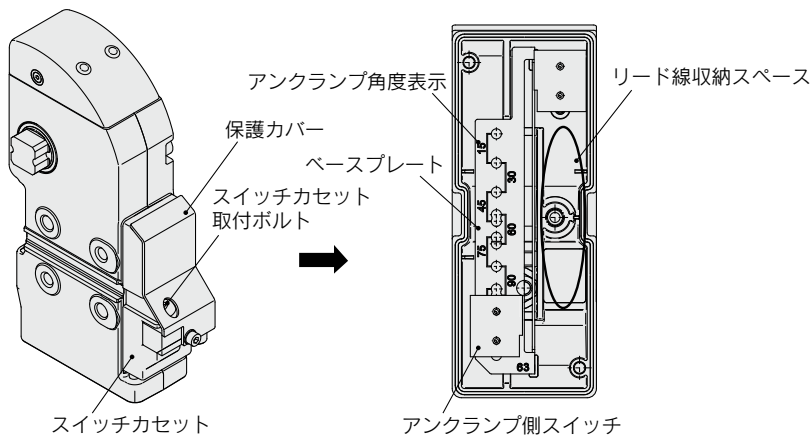
スイッチカセット取付ボルト締付トルク
