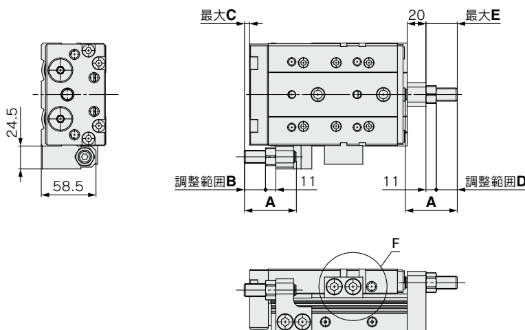
詳細図F:前進端アジャストブロック取付位置
