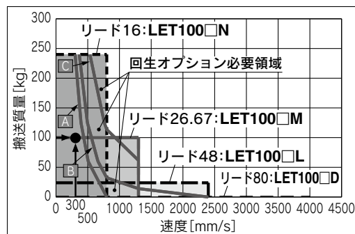
〈速度－搬送質量グラフ〉 (LET100)
