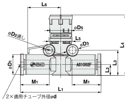
右側面図
