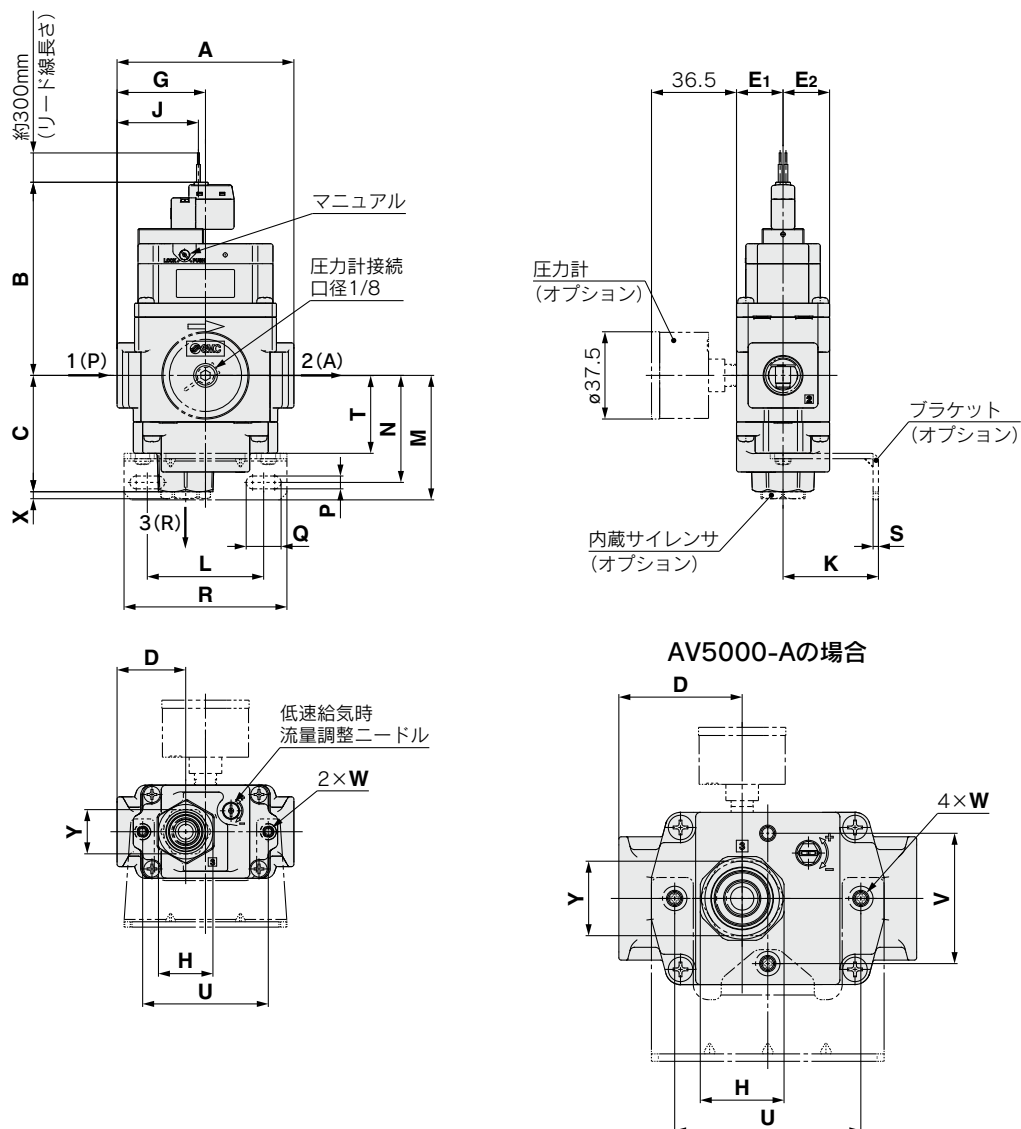
寸法表
