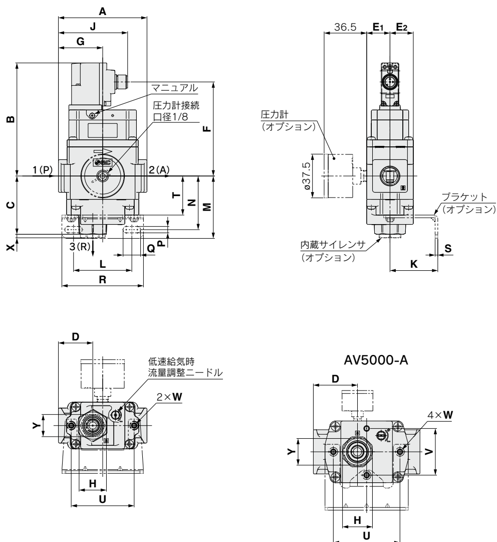
寸法表
