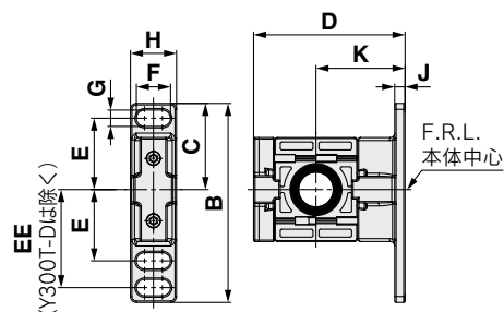
ブラケット付スペーサ(標準)
