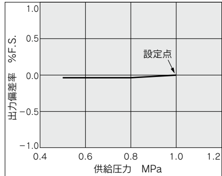
圧力特性
