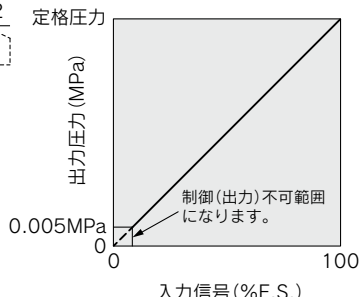
図1.入出力関係図
