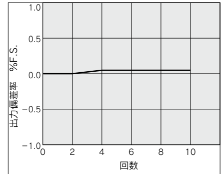
繰返し性
