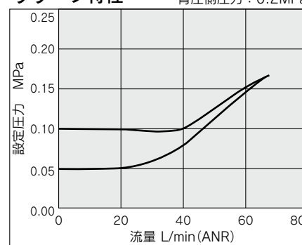
リリーフ特性
