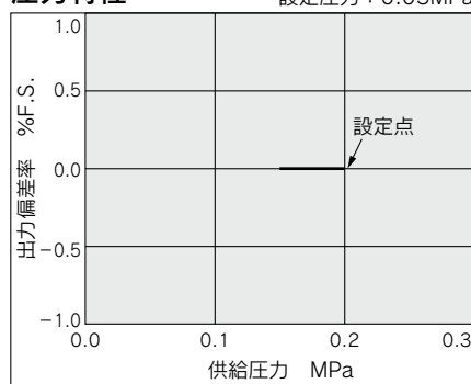
圧力特性
