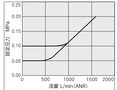
リリーフ特性
