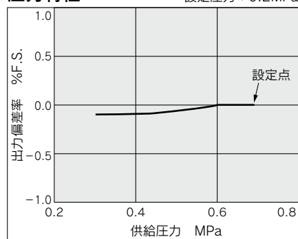
圧力特性
