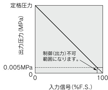
入出力特性図
