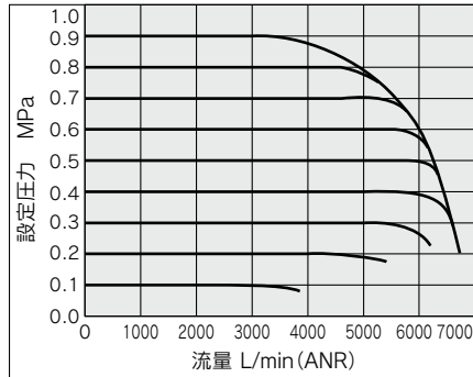
流量特性
