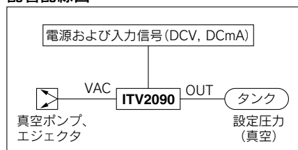
配管配線図
