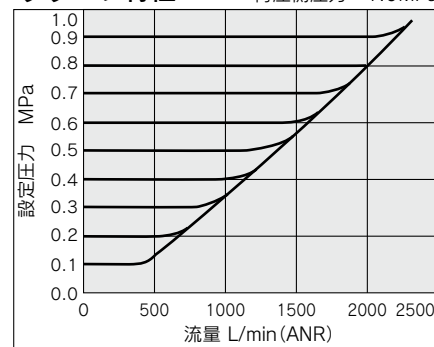
リリーフ特性
