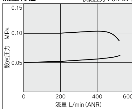
流量特性
