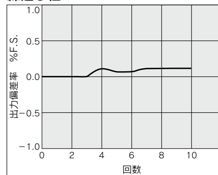
繰返し性
