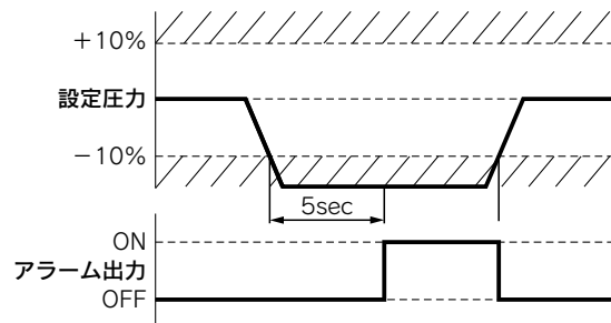
図2 出力圧力とアラーム出力の関係
