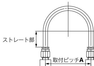
図1 推奨配管図
