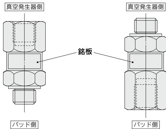
図1.取付方向
