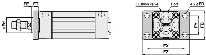
Rod Flange
