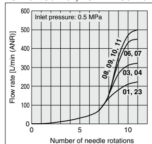
AS2□01FSG□-02, AS2□11FSG□-02
