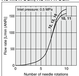
AS4□01FSG□, AS4□11FSG□
