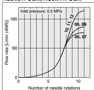
AS3□01FSG□, AS3□11FSG□
