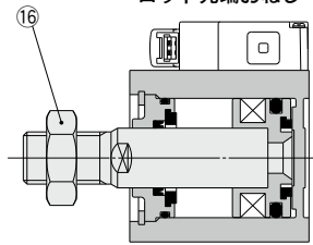
ロッド先端おねじ
