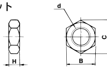
材質：炭素鋼 (mm)
