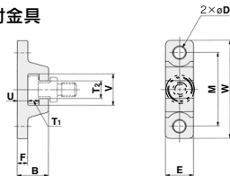
材質：クロムモリブテン鋼 (ニッケルめっき) (mm)
