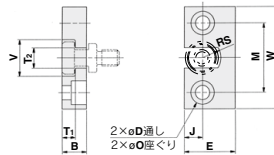
材質：炭素鋼 (ニッケルめっき) (mm)
