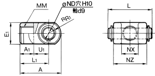
材質：鋳鉄 (mm)
