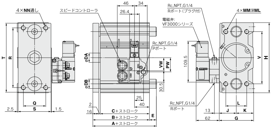
MVGQM,MVGQL共通寸法表
