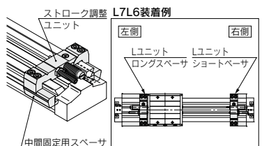
ストローク調整ユニット装着図
