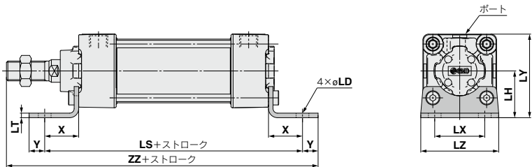
軸方向フート形 (mm)
