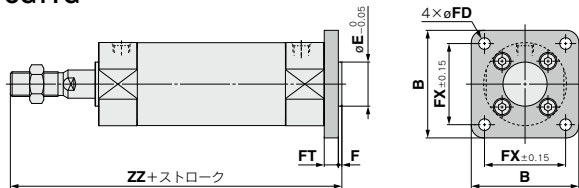
フランジ形 (mm)
