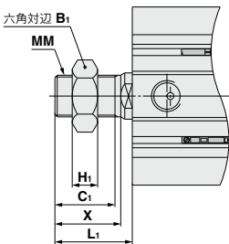
ロッド先端ねじ
