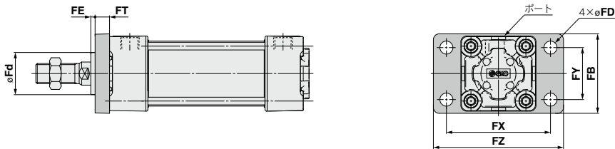
ロッド側フランジ形 (mm)
