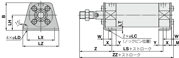
軸方向フート形 (mm)
