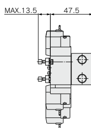
絞り弁内蔵タイプ
