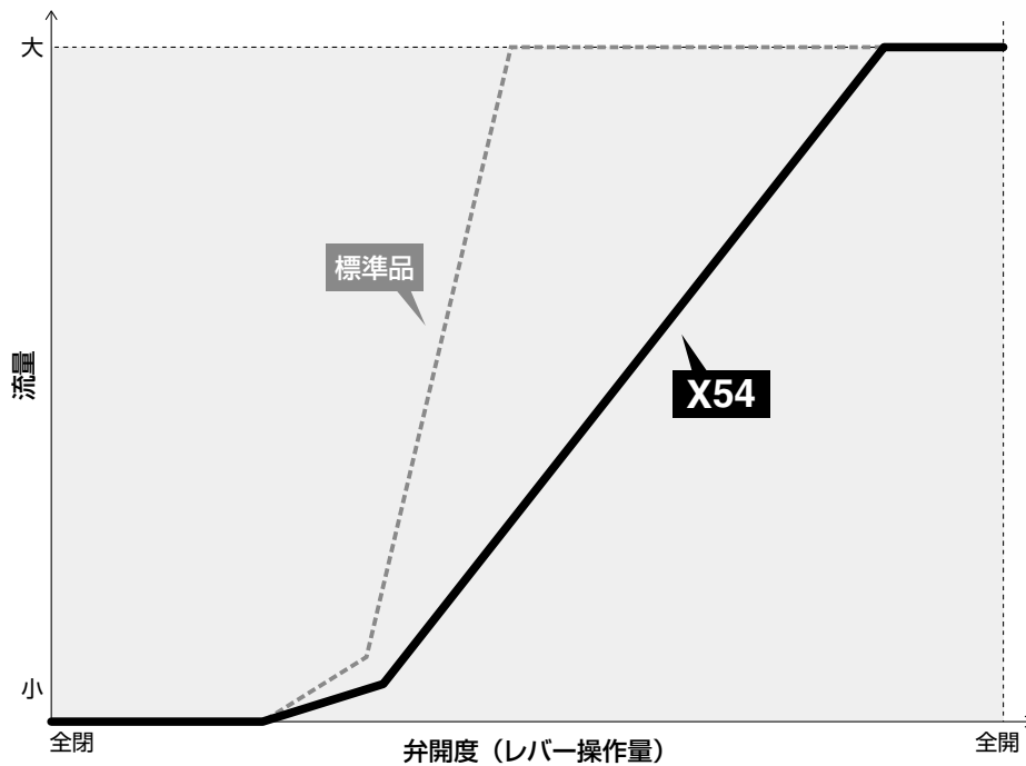
レバー操作量と流量の関係(イメージ)
