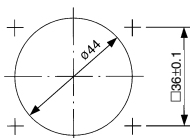
パネル取付穴 (ソケット側カバー付)
