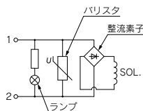
サージ電圧保護回路・ランプ付
