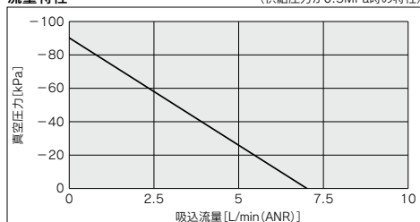
流量特性
