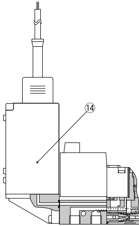
単体／真空用圧カスイッチ仕様
