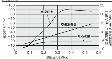
排気特性
